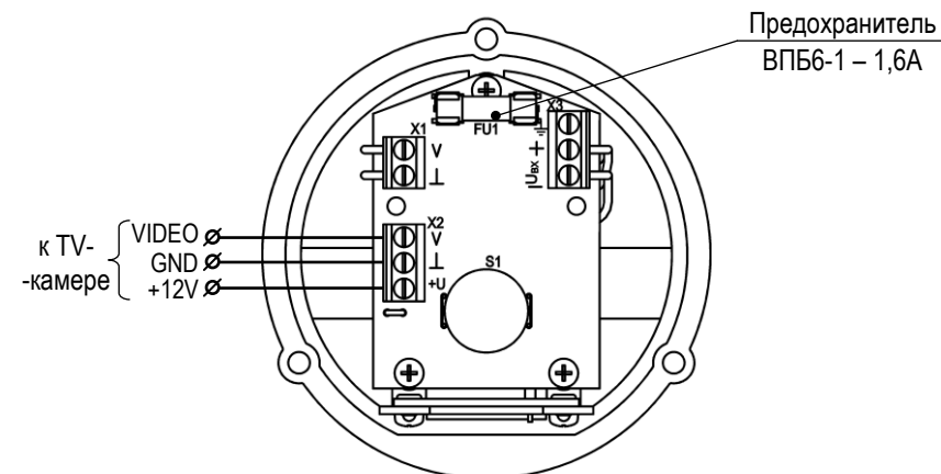
Рис.2 Подключение ТГБ-5-180-~24/12 и ТГБ-5А-180-~24/12
