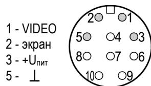
Рис.4 Распайка розетки РС-10 (вид со стороны распайки проводников)
