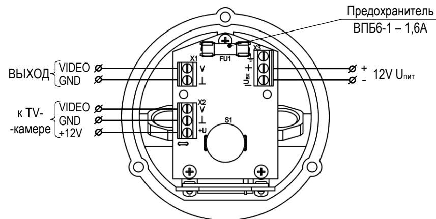
Рис.1 Подключение ТГБ-5-180-12/12
