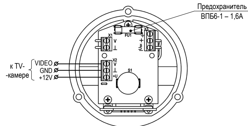
Рис.3 Подключение ТГБ-5-180-24/12 и ТГБ-5А-180-24/12
