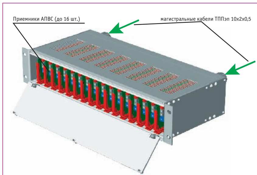
Рис. 4. Крейт 2U19-16
