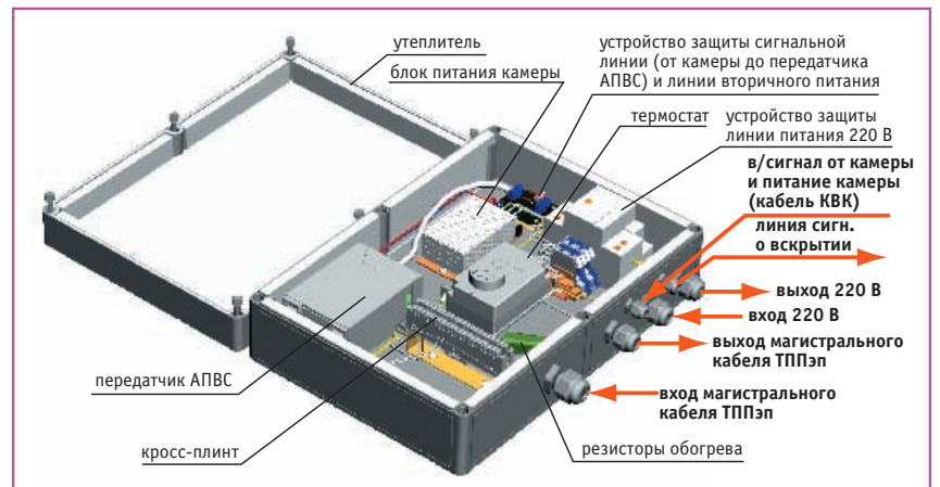
Рис. 2. Монтажная обогреваемая гермокоробка КМГО
